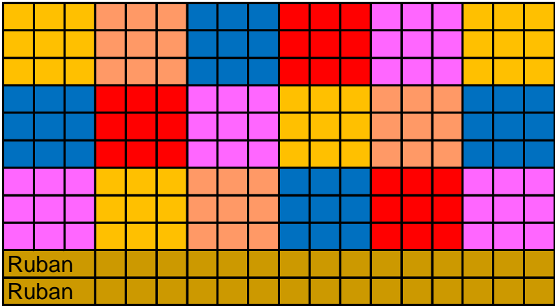
Le DAMIER :
