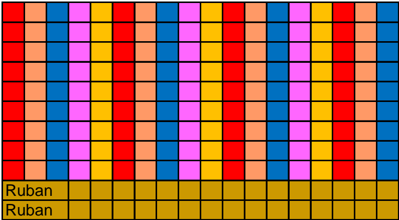
Les RAYURES :
